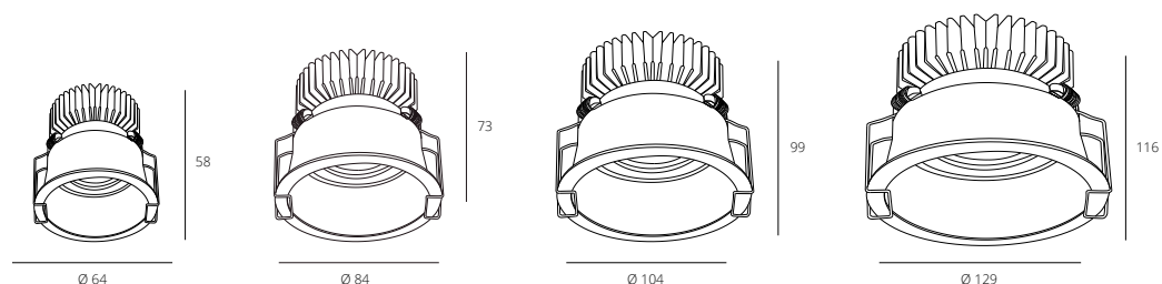
RSL74W005-2 /7W
