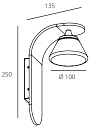
RWLB175/7W
