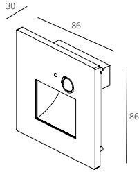
RWLB180/1W
