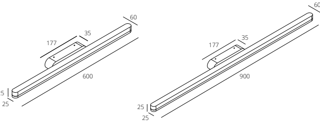
RWLB115/13W
