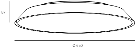
RXD4002/60W
