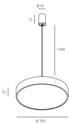
RHL73029/30W
