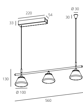
RHL77026/3x6W
