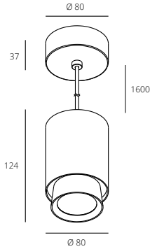
RHL7778/15W
