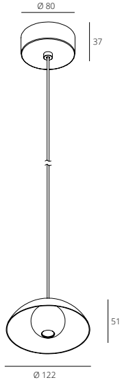
RHL7755/5W
