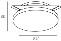
RDL74016-3/3W
