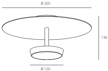
RXD4003/12W
